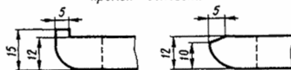
Черт 96. Подкладка КД65 (К4-65)
