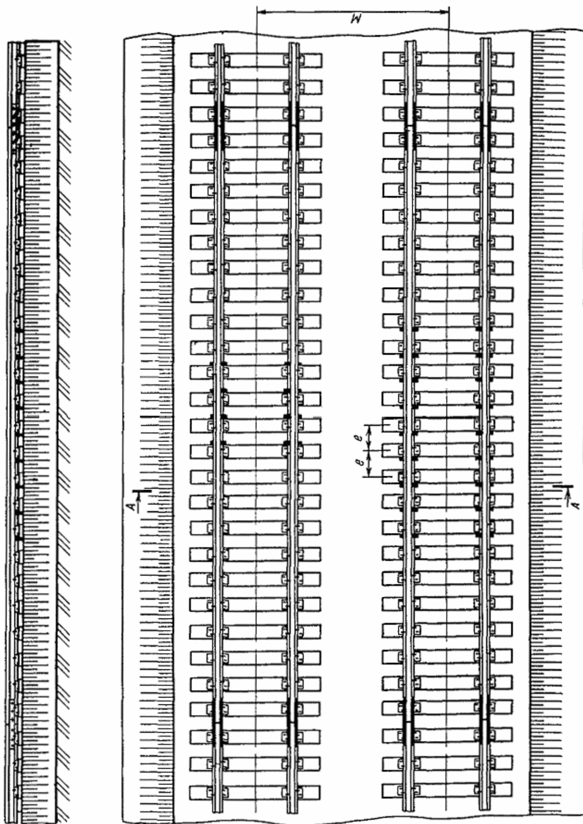
Черт. 1. Верхнее строение пути с деревянными шпалами в прямых участках:
