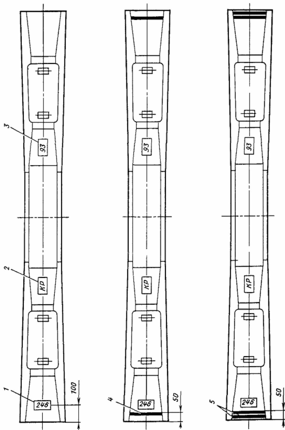
Черт. 23. Маркировка железобетонных шпал:
