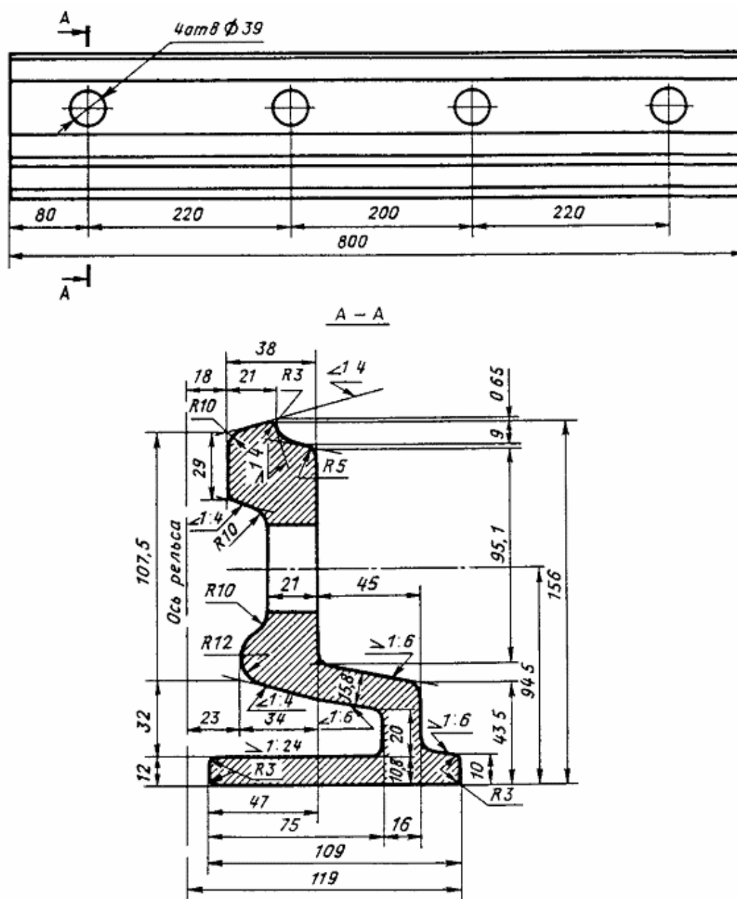
Черт. 140. Накладка объемлющая НИ-65
