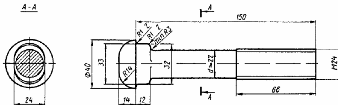
Черт. 54. Болт путевой 24×150 по ГОСТ 11530-76 для рельсов типа Р50
