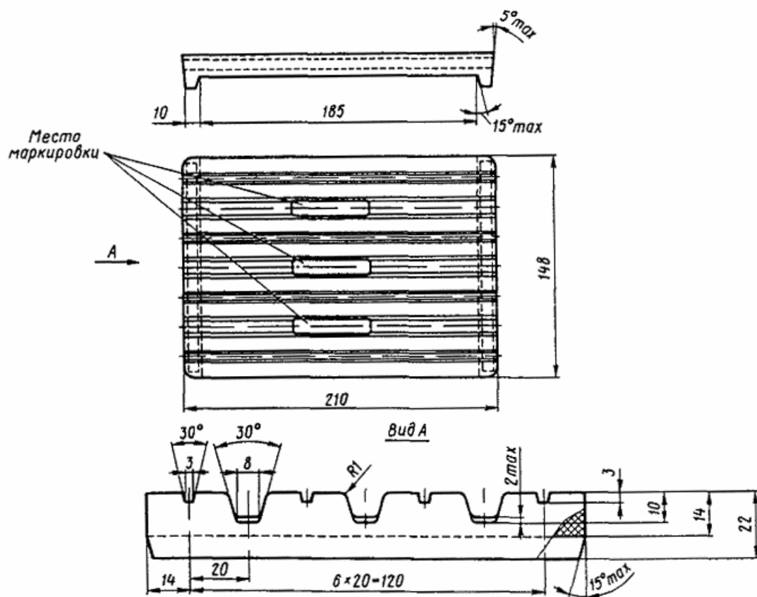
Черт. 113. Прокладка ЖБР
