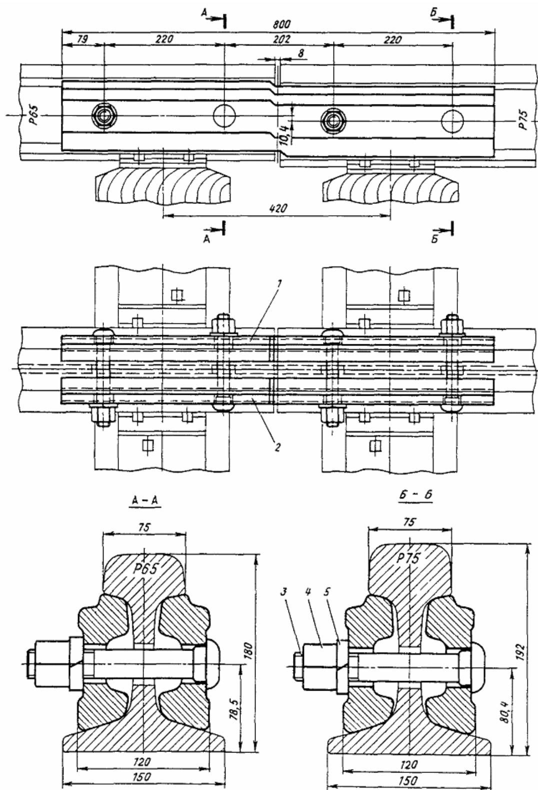
Черт. 115. Переходный стык рельсов Р75 - Р65
