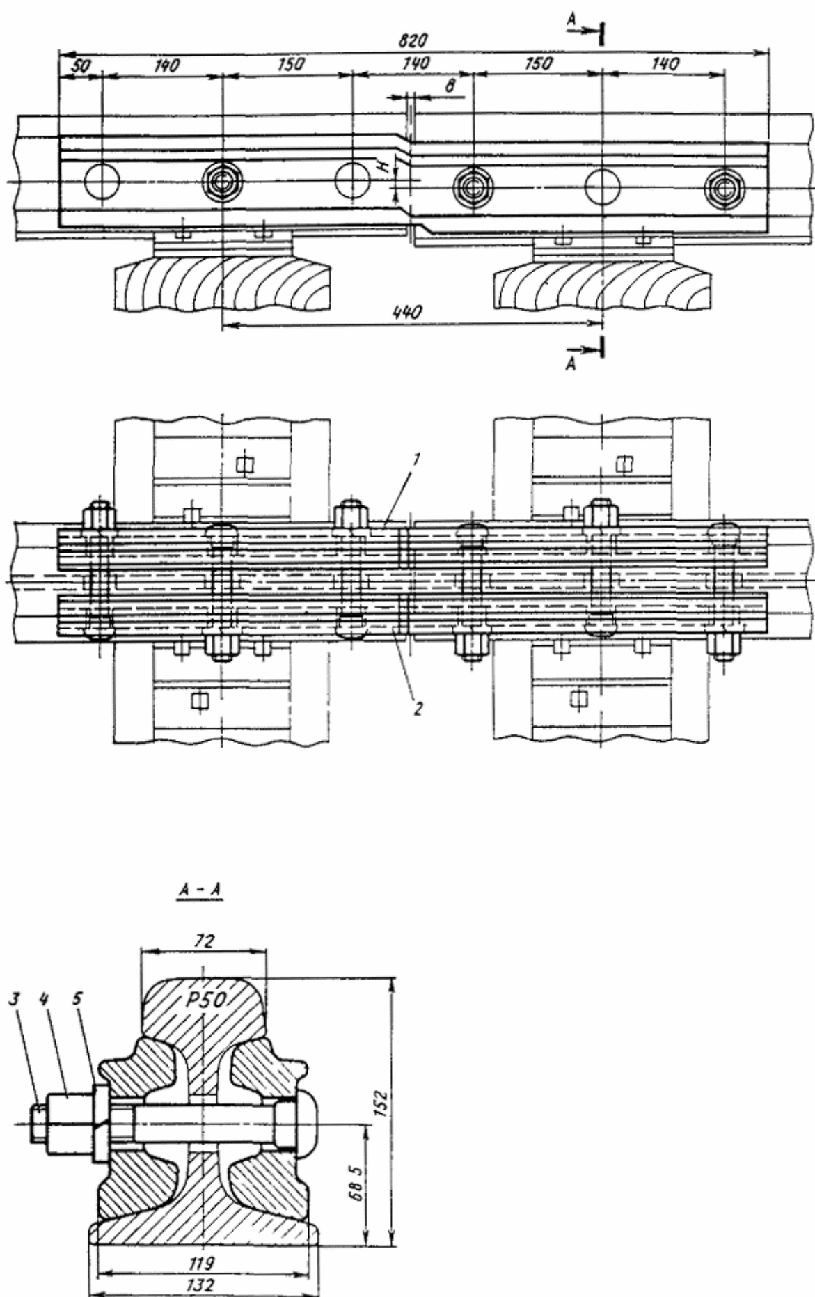
Черт. 124. Переходный стык рельсов P50 - P50
