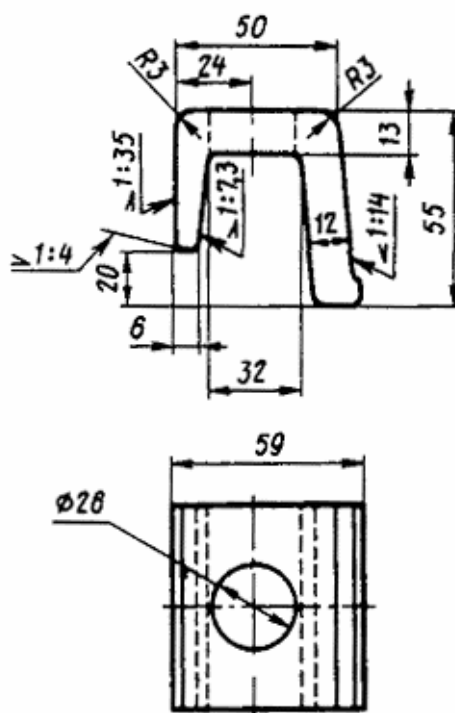
Черт. 91. Клемма раздельного рельсового скрепления (СК) по ГОСТ 22343-77
