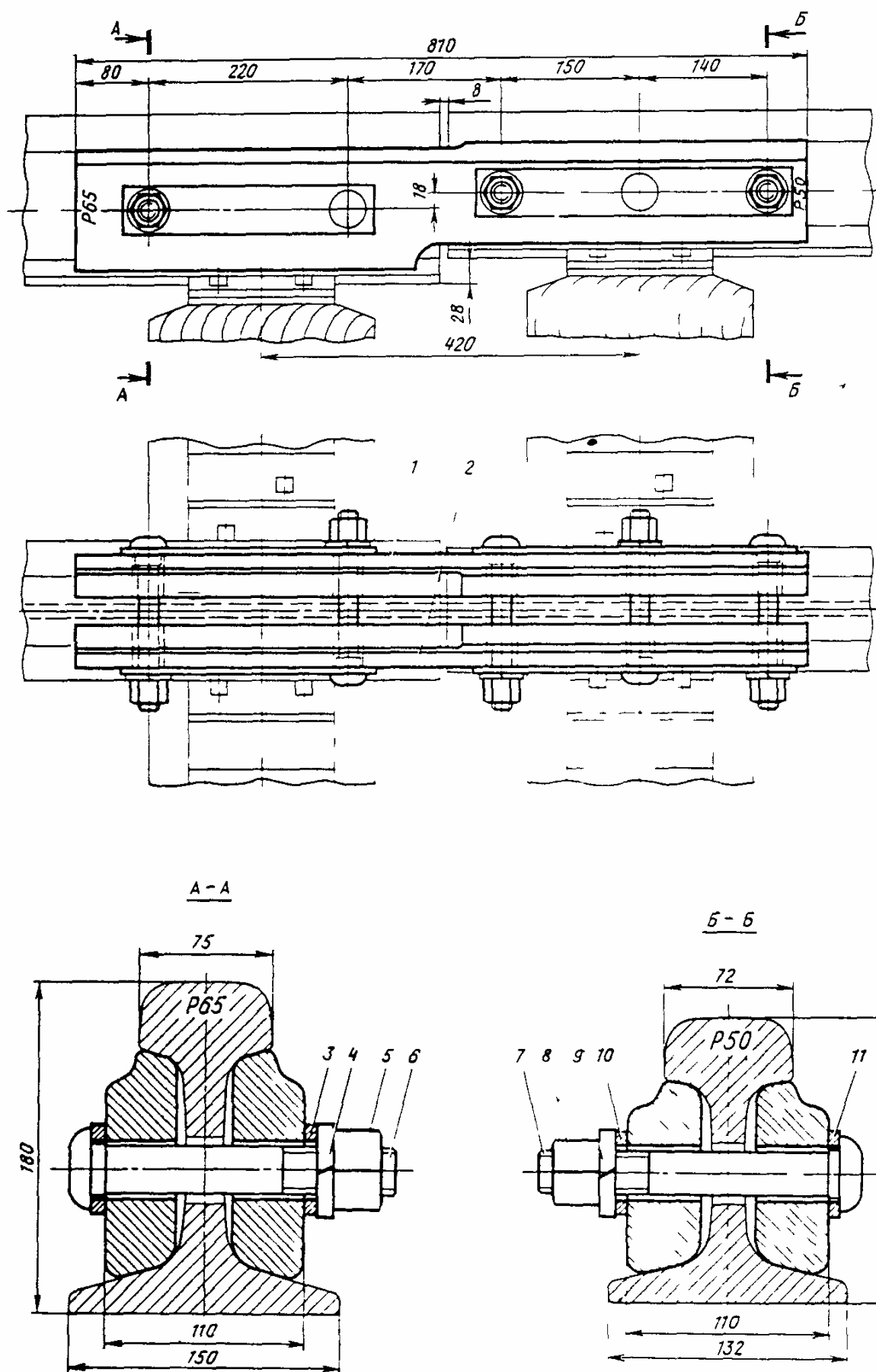
Черт. 121. Переходный стык рельсов Р65 - Р50 на переходных накладках из полосы
