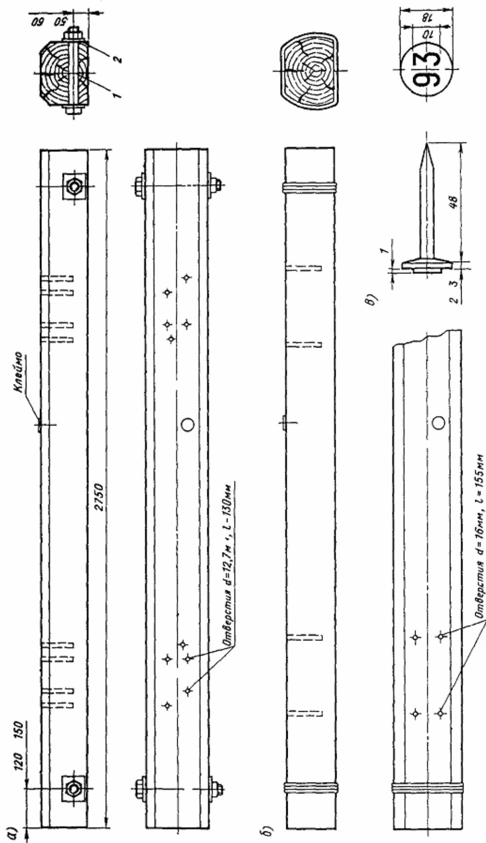
Черт. 14. Шпала деревянная
