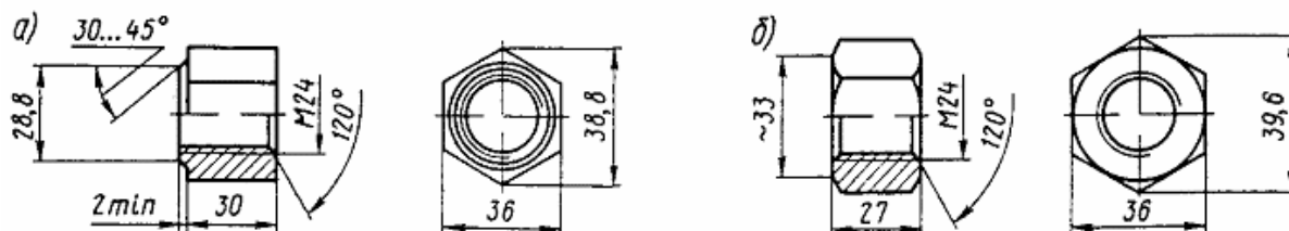
Черт. 55. Гайка М24 по ГОСТ 11532-76 к болтам для рельсов типа Р50:
