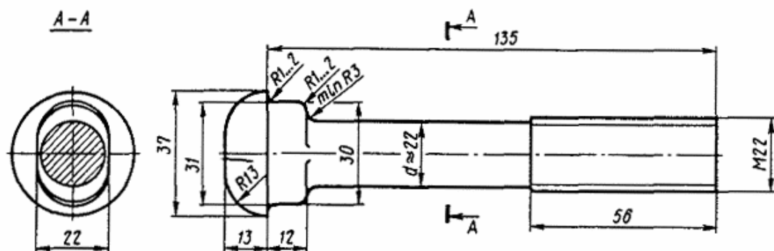
Черт. 56. Болт путевой M22×135 по ГОСТ 11530-76 для рельсов типов Р43, Р38 и I-а
