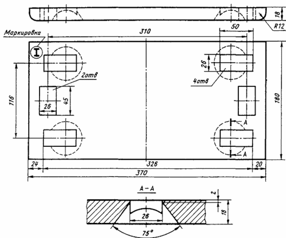
Черт. 172. Подкладка для рельсов типа Р50
