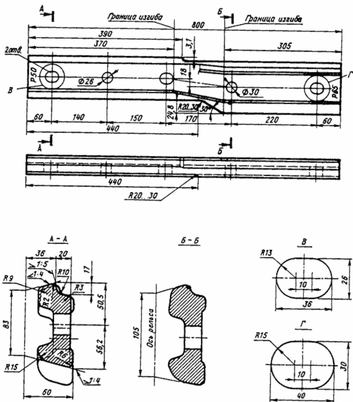
Черт. 119. Накладка переходная Р65 - Р50 (правая)
