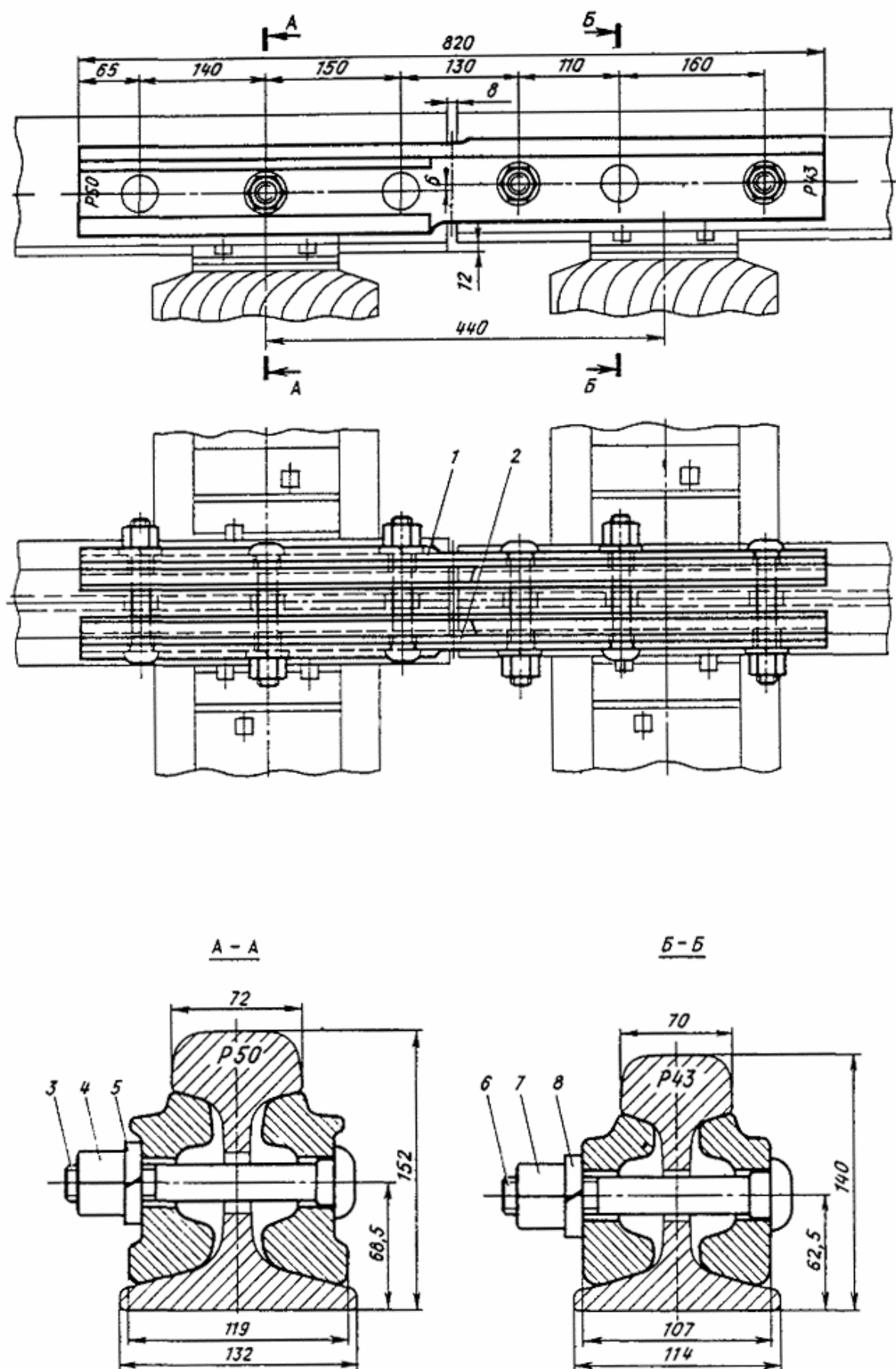
Черт. 127. Переходный стык рельсов Р50 - Р43
