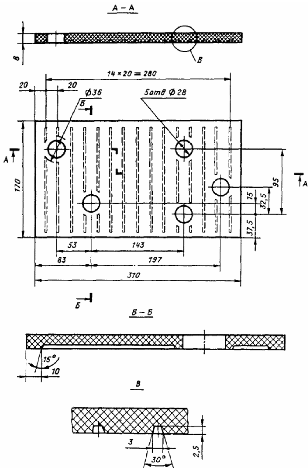
Черт. 69. Прокладка под подкладку Д50
