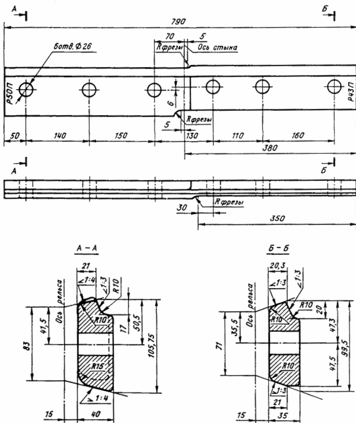
Черт. 131. Накладка переходная Р50 - Р43 из полосы (правая)
