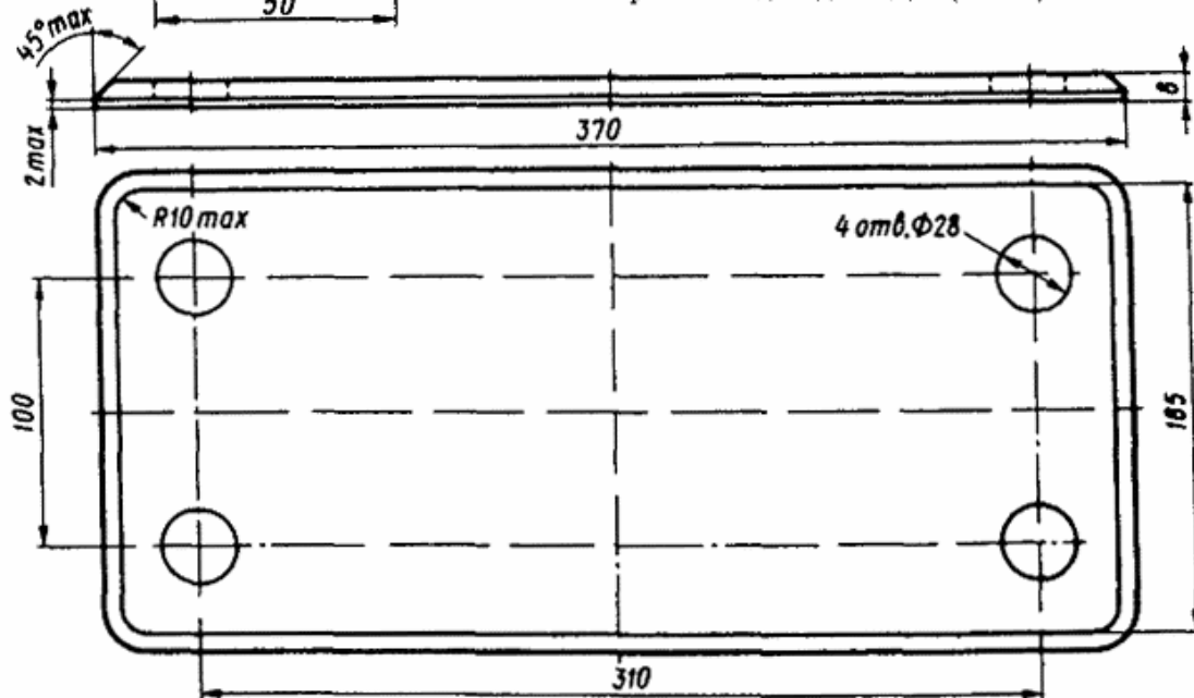
Черт. 97. Прокладка под подкладку КД65
