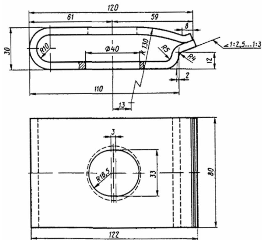
Черт. 111. Клемма стыковая ЖБР
