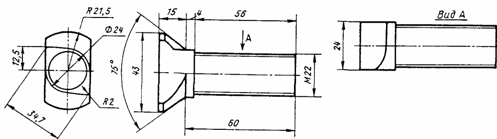
Черт. 174. Болт М22х60
