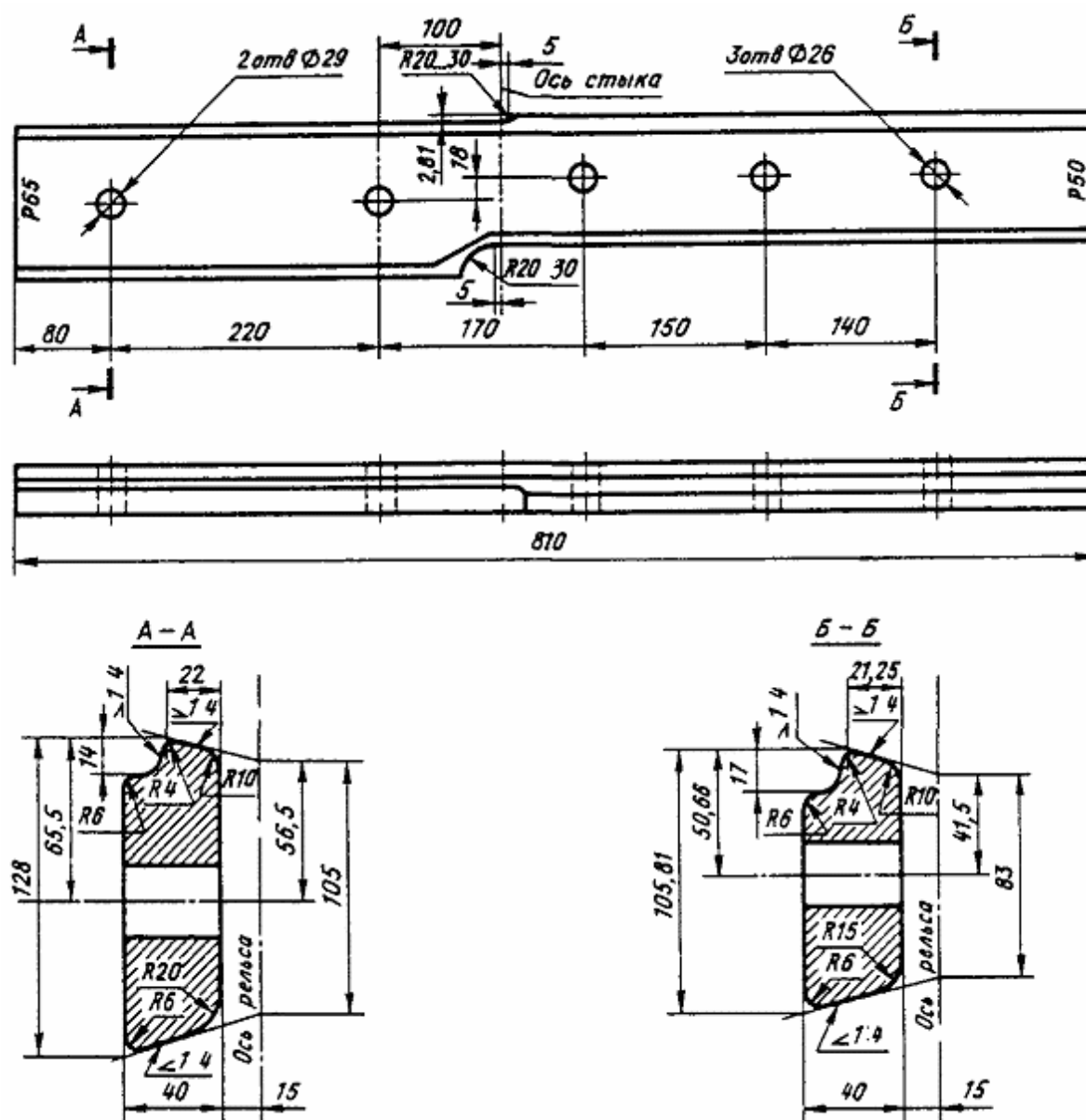
Черт. 123. Накладка переходная Р65 - Р50 из полосы (левая)
