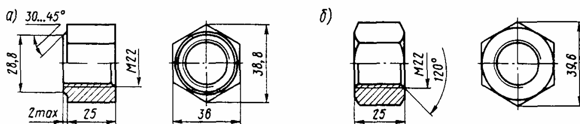
Черт. 57. Гайка M22 по ГОСТ 11532-76 к болтам для рельсов типов Р43, Р38, I-а и Р33:
