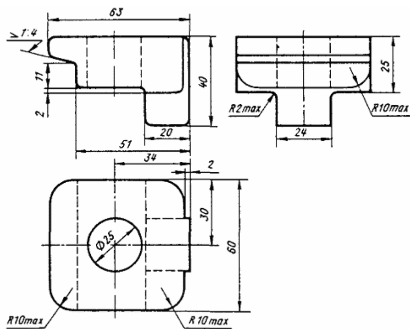
Черт. 173. Клемма КС
