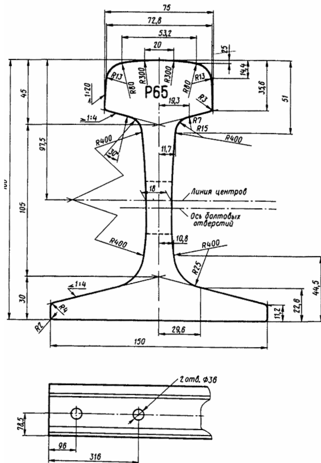
Черт. 30. Рельс типа Р65 по ГОСТ 8161-63 (Рельсы поставлялись в период 1964 - 1975 гг.)
