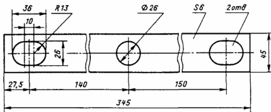
Черт. 155. Планка под болты ППБ-50
