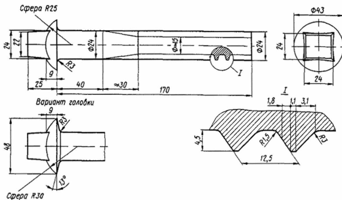
Черт. 98. Шуруп путевой 24×170 по ГОСТ 809-71
