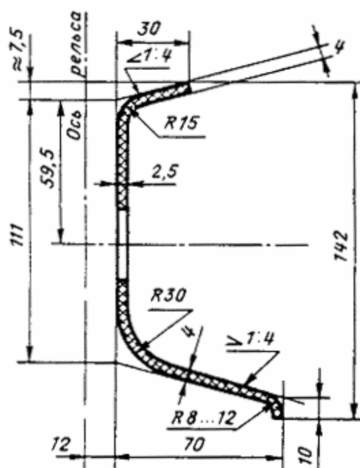
Черт. 141. Прокладка боковая составная ПБС-65
