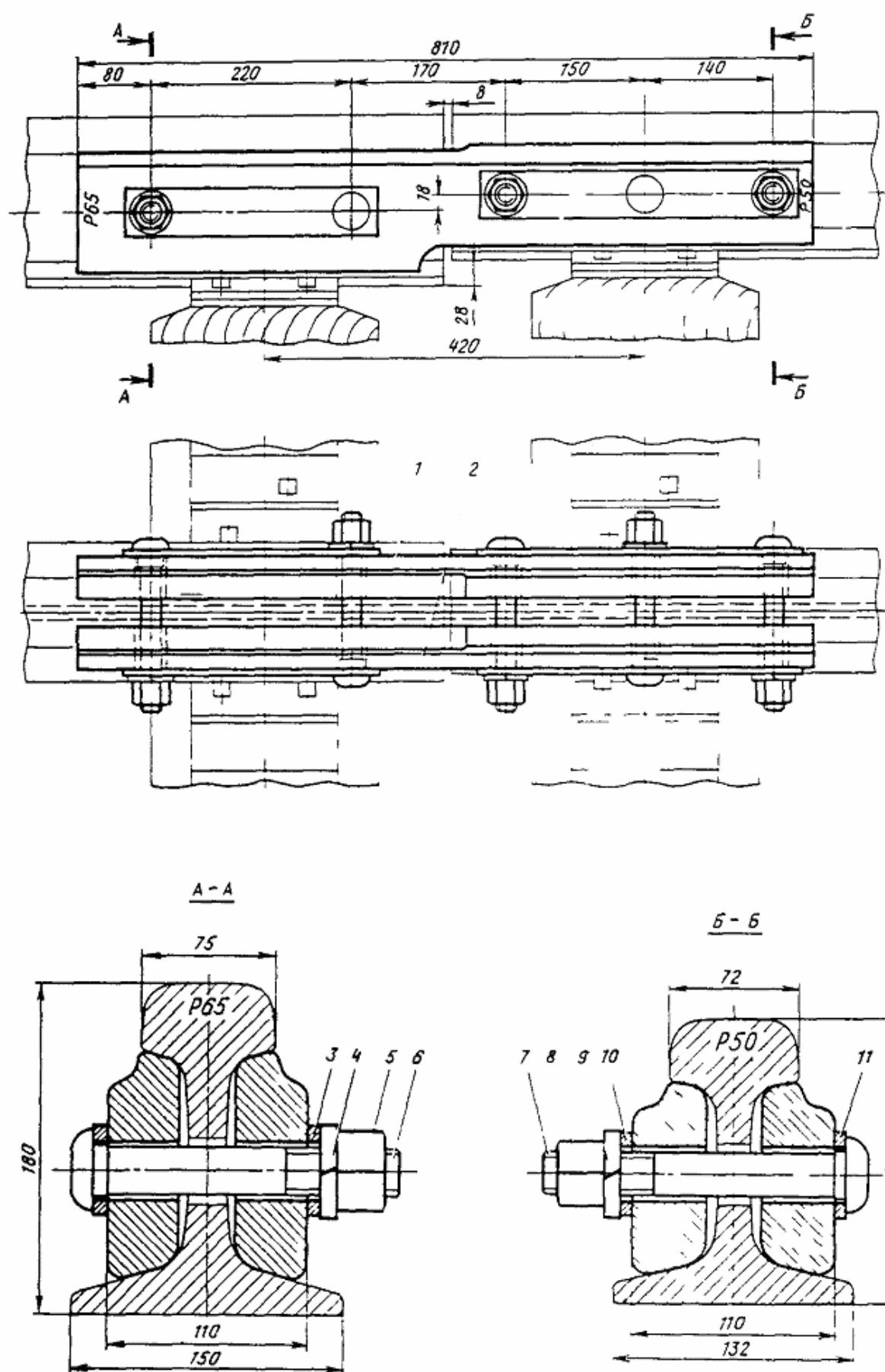
Черт. 120. Накладка переходная P65 - P50 (левая)
