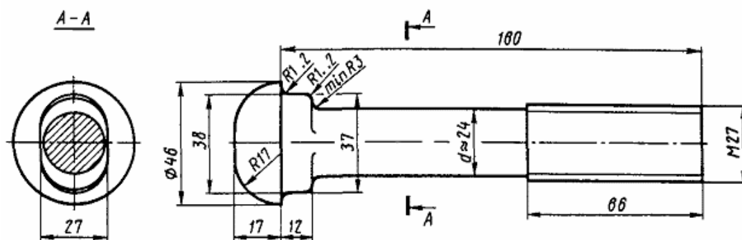
Черт. 52. Болт путевой М27×160 по ГОСТ 11530-76 для рельсов типов Р65 и Р75
