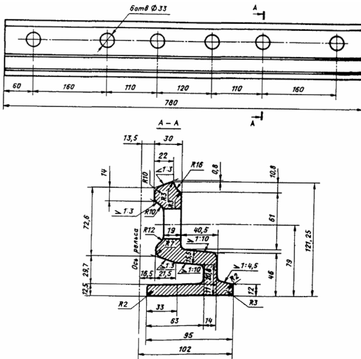
Черт. 160. Накладка объемлющая НИ-43
