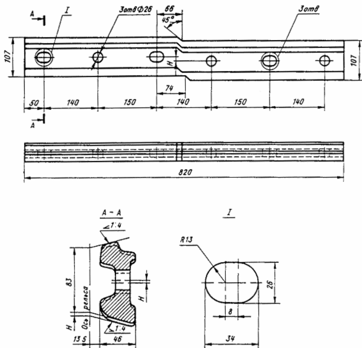
Черт. 125. Накладка переходная Р50 - Р50 (правая) (Величина перегиба H должна соответствовать вертикальному износу головки рельса)
