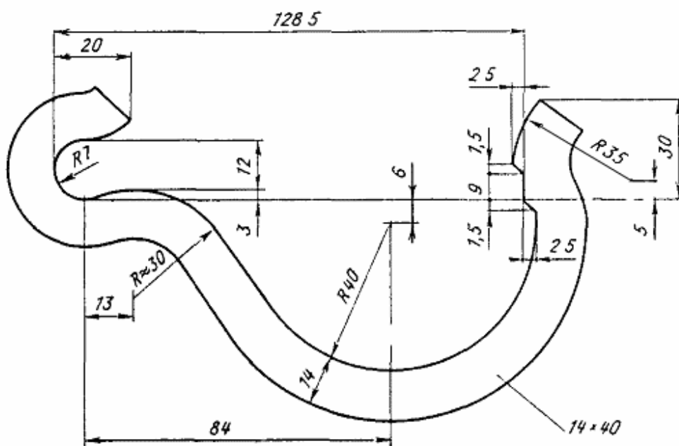
Черт. 76. Противоугол пружинный ПШ1-50 к рельсам типа Р50
