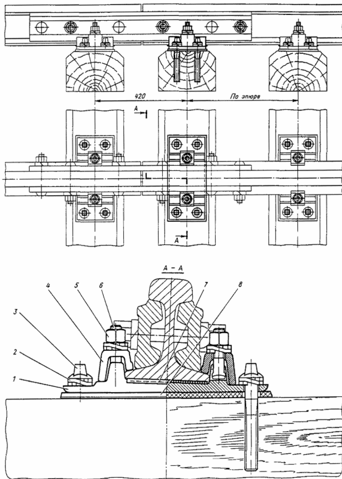
Черт. 95. Рельсовое крепление КД65 (К4-65) на деревянных шпалах с рельсами типов Р65 и Р75
