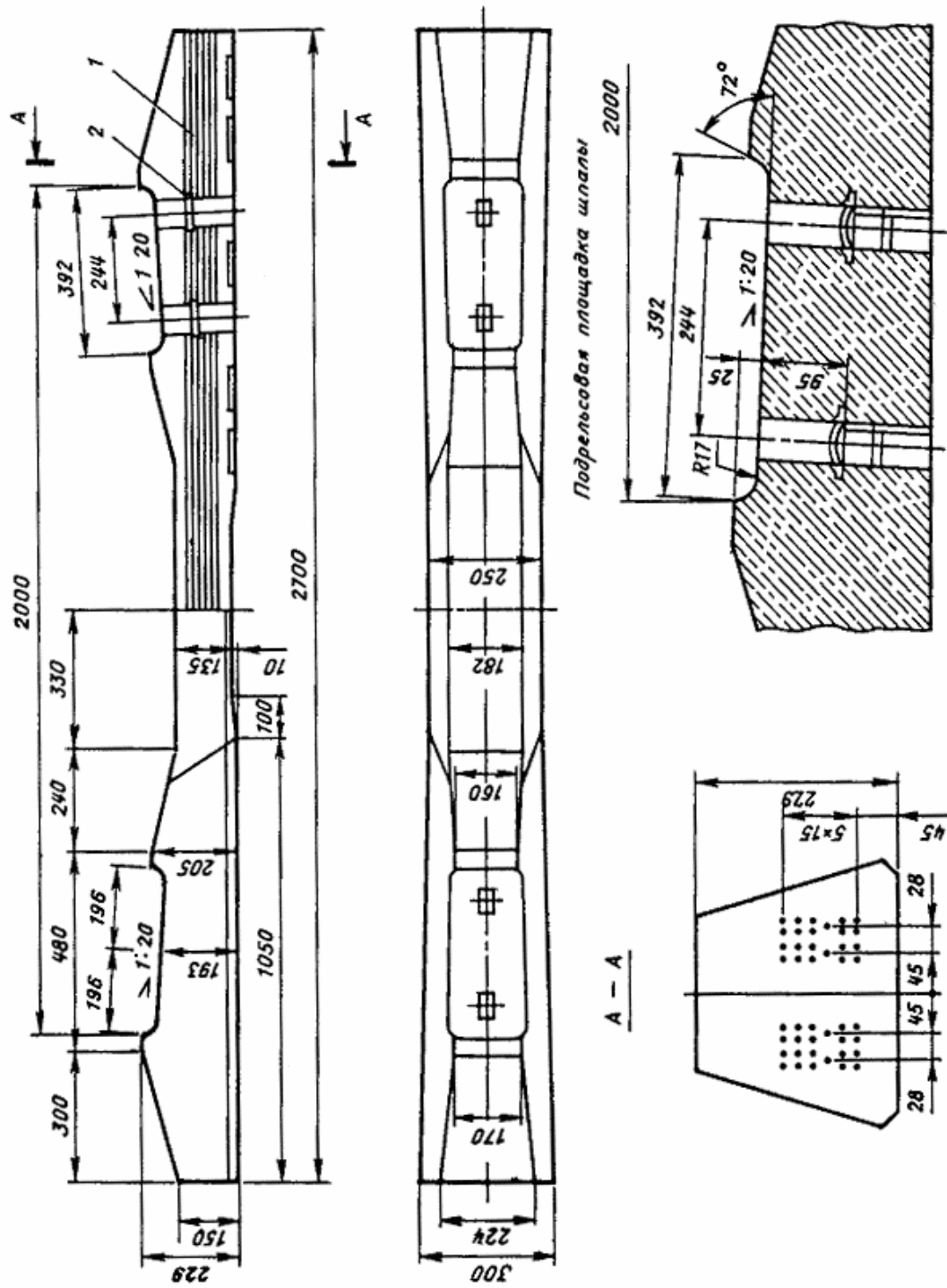
Черт. 19. Шпала железобетонная типа ШС-2у по ГОСТ 10629-78:
