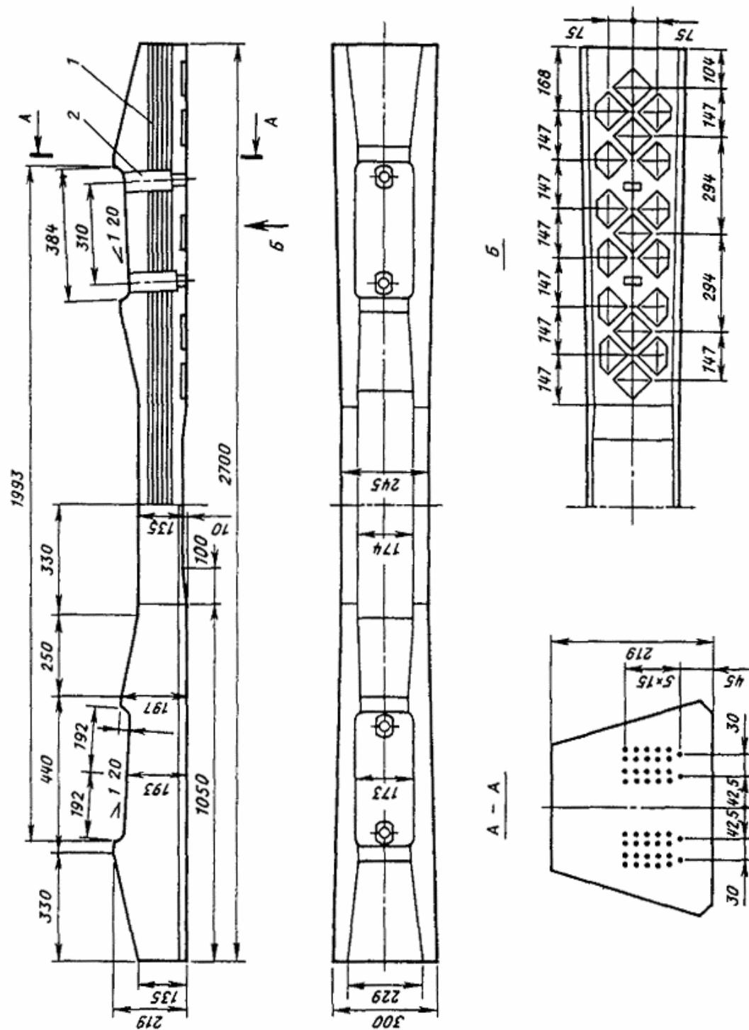
Черт. 17. Шпала железобетонная типа С-56-1 по ГОСТ 10629-63:
