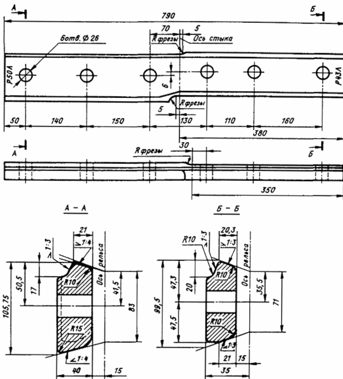
Черт. 132. Накладка переходная P50 - P43 из полосы (левая)
