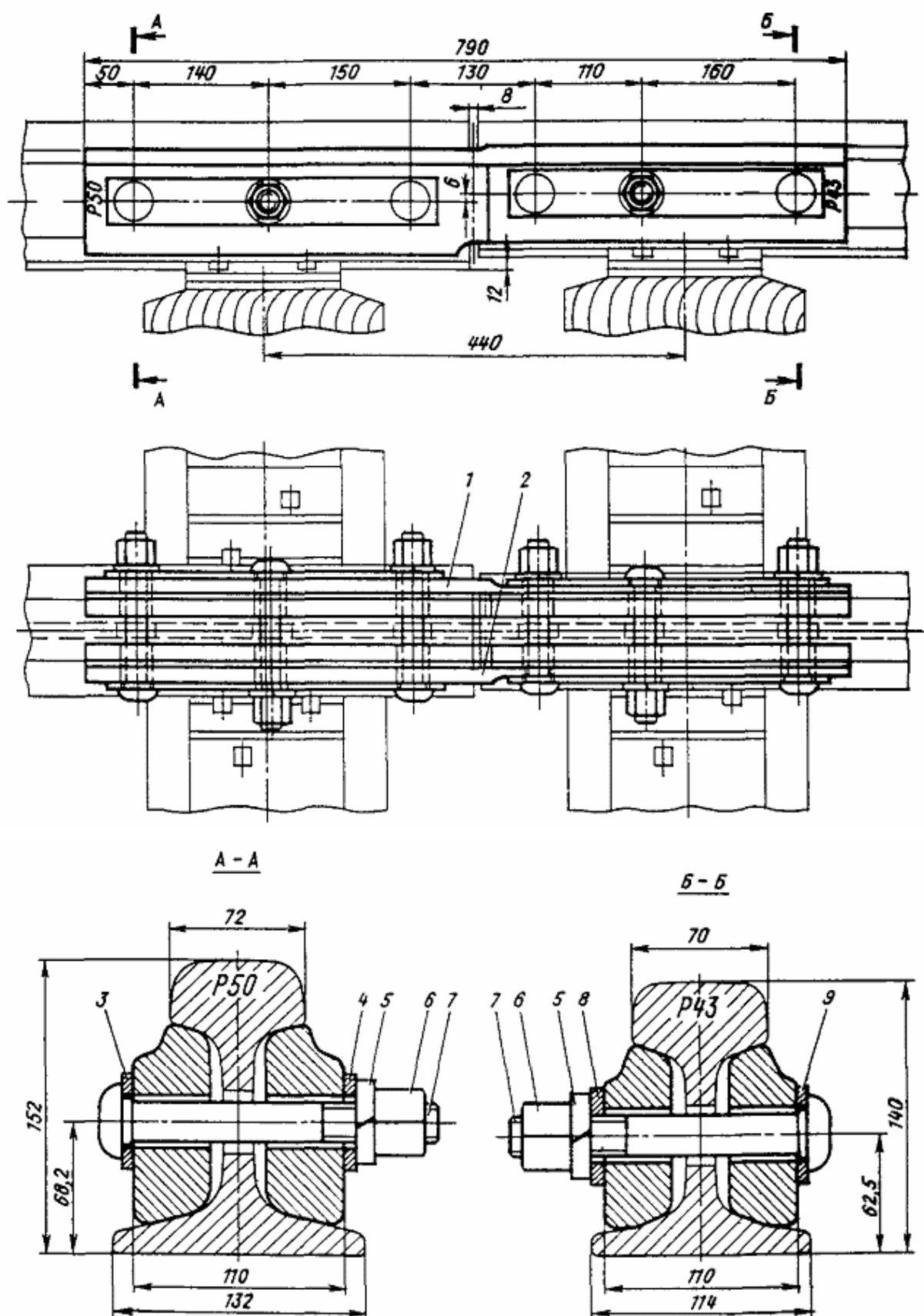
Черт. 130. Переходный стык рельсов Р50 - Р43 на переходных накладках из полосы
