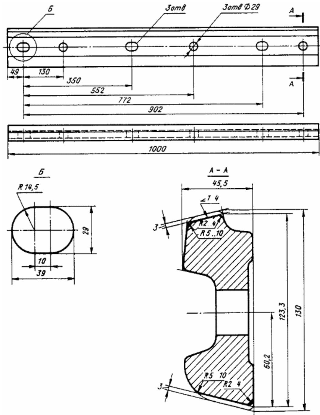
Черт. 136. Накладка двухголовая строганая типа Р65
