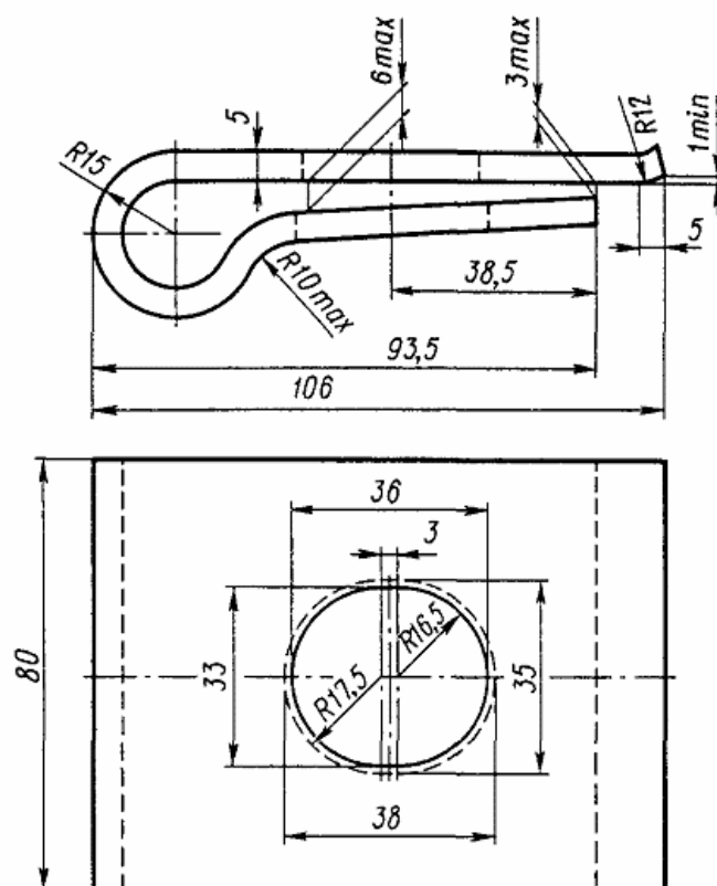
Черт. 108. Клемма стыковая АС14
