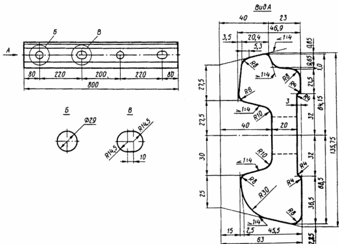
Черт. 47. Накладка двухголовая к рельсам типа Р75 по проекту 751/ЦП
