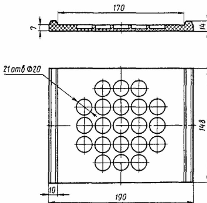
Черт. 99. Прокладка под подошву рельсов Р65 в креплении КД65
