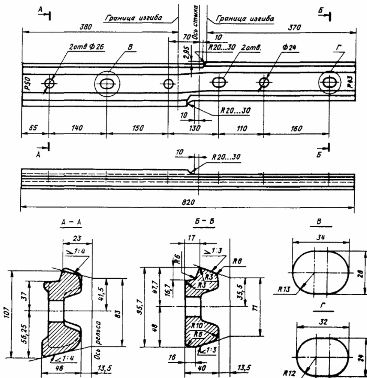
Черт. 129. Накладка переходная P50 - P43 (левая)
