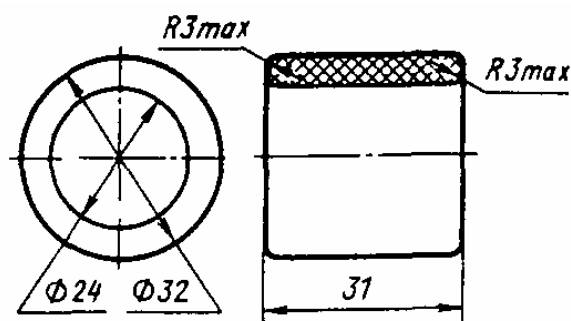
Черт. 168. Втулка В-22
