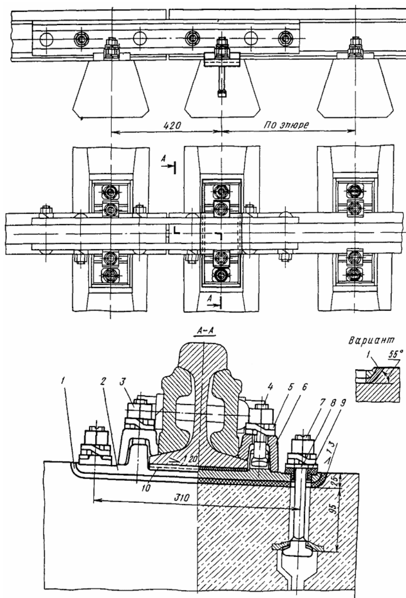
Черт. 77. Рельсовое скрепление КБ65 на железобетонных шпалах с рельсами типов Р65 и Р75
