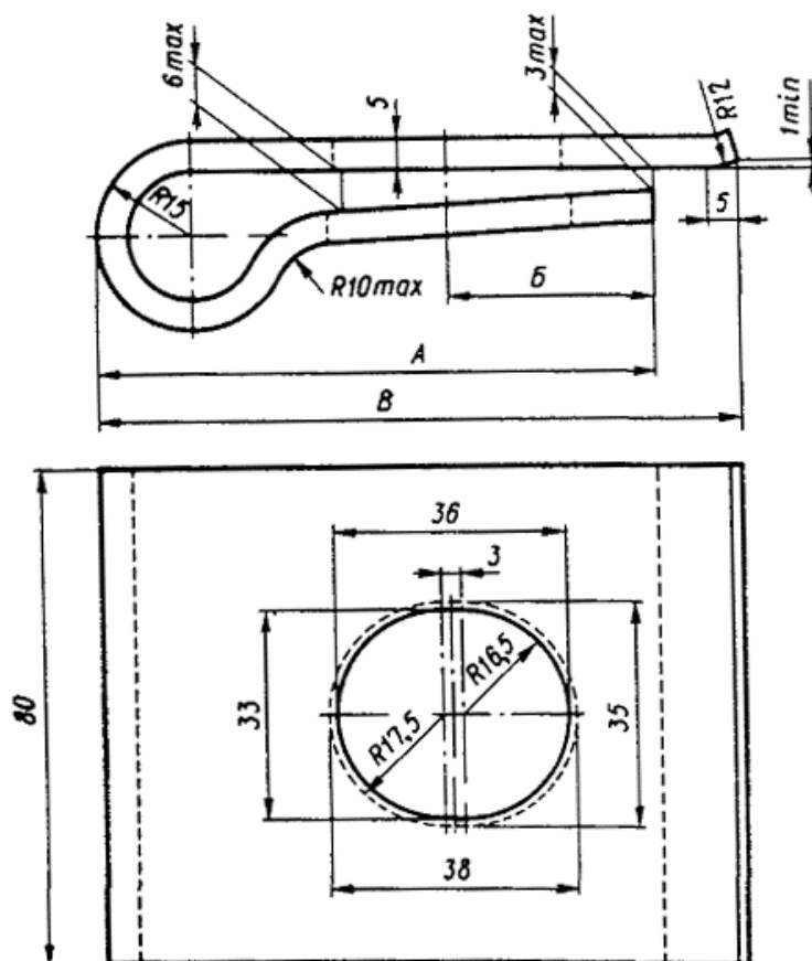
Черт. 102. Клемма стыковая АС10 и АС12
