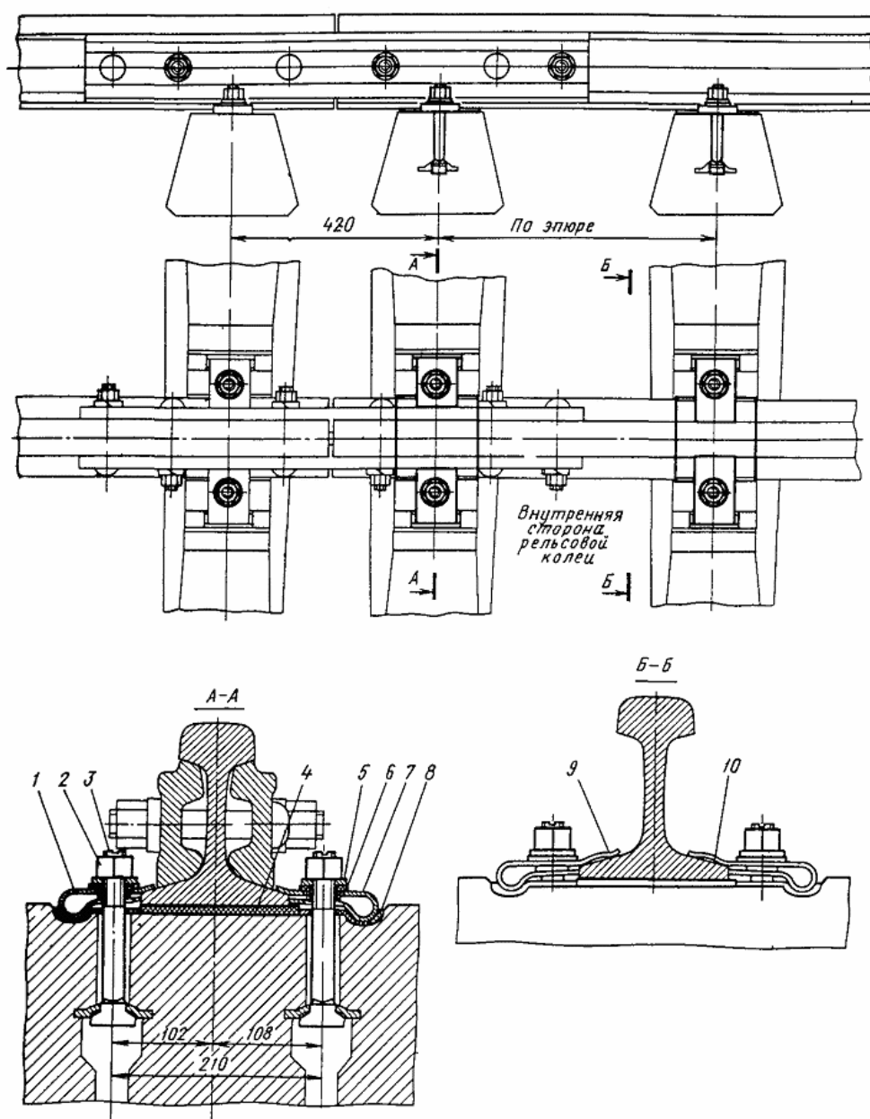
Черт. 100. Рельсовое крепление ЖБ65 на железобетонных шпалах с рельсами типов Р65 и Р75
