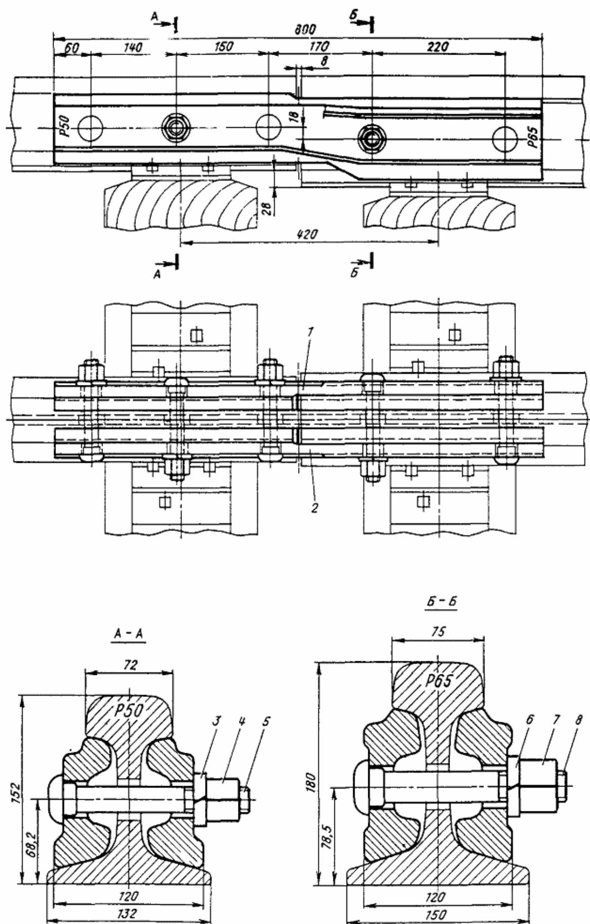
Черт. 118. Переходный стык рельсов Р65 - Р50
