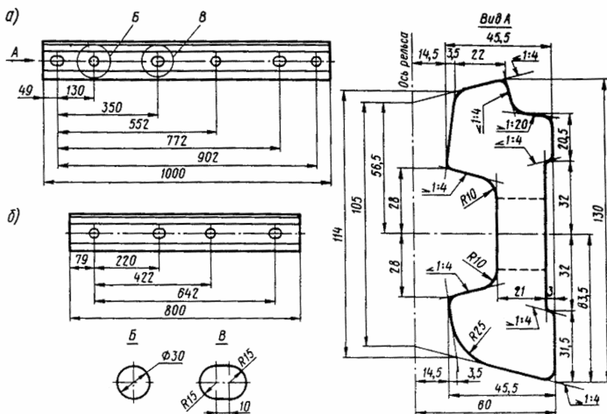
Черт. 46. Накладка двухголовая к рельсам типов P75, P65 по ГОСТ 8193-73:
