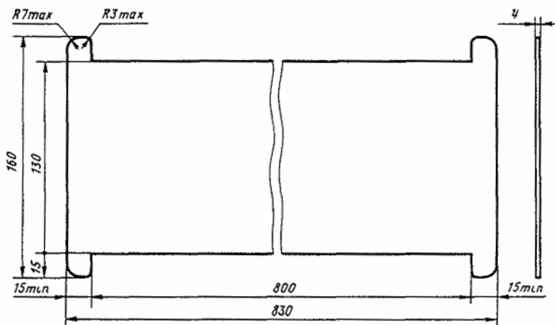
Черт. 166. Прокладка нижняя ПН-43
