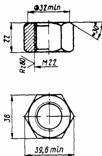
Черт. 81. Гайка М22×22 по ГОСТ 16018-79
