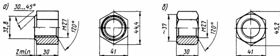
Черт. 53. Гайка М27 по ГОСТ 11532-76 к болтам для рельсов типов Р65 и Р75:
