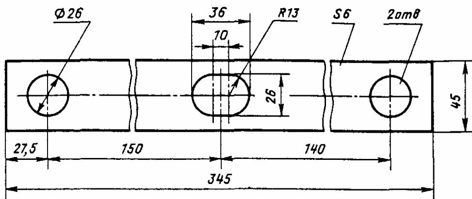
Черт. 154. Планка стопорная СИ-50-2
