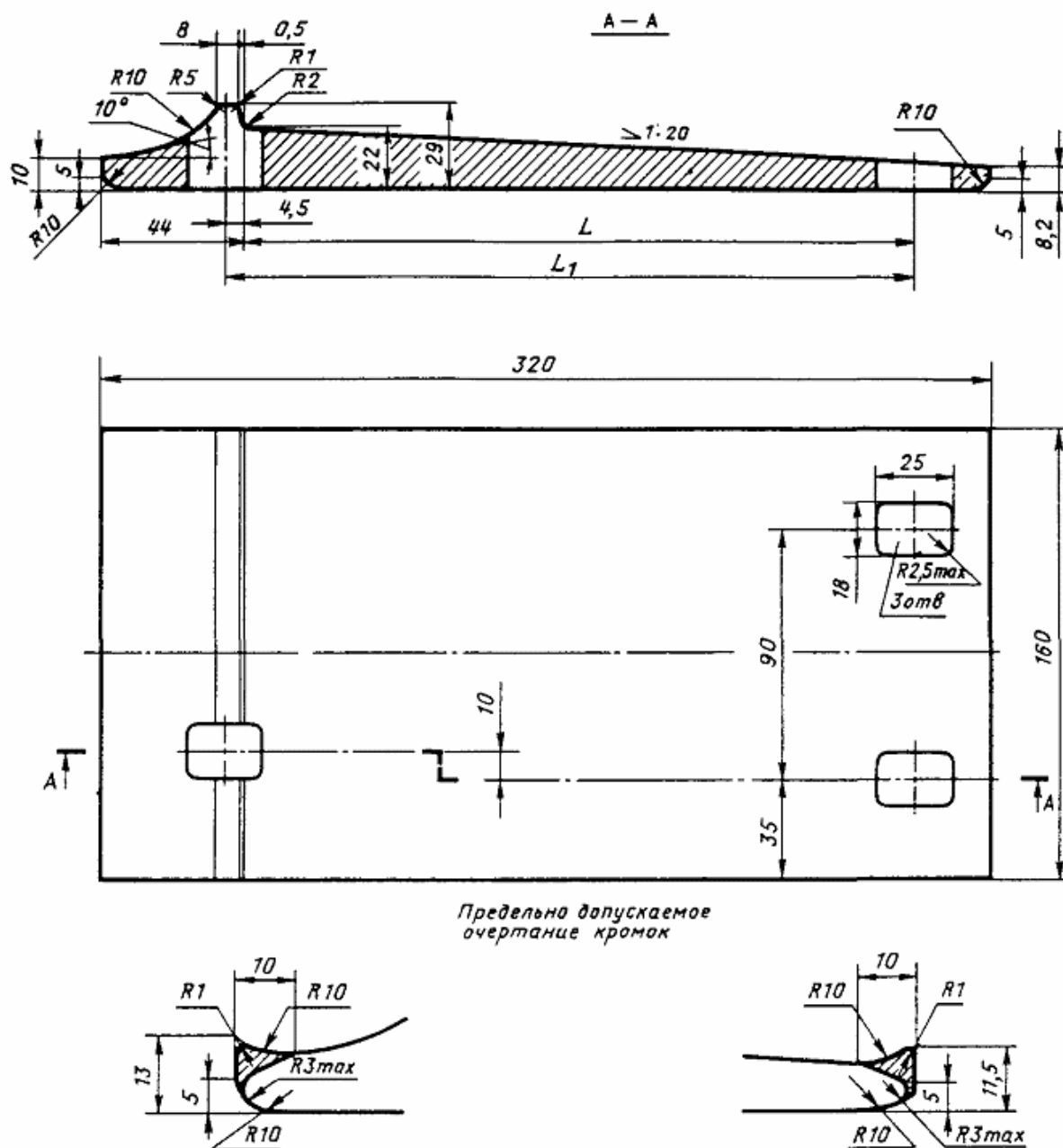
Черт. 143. Подкладки ПИ-65, ПИ-50, ПИ-43
