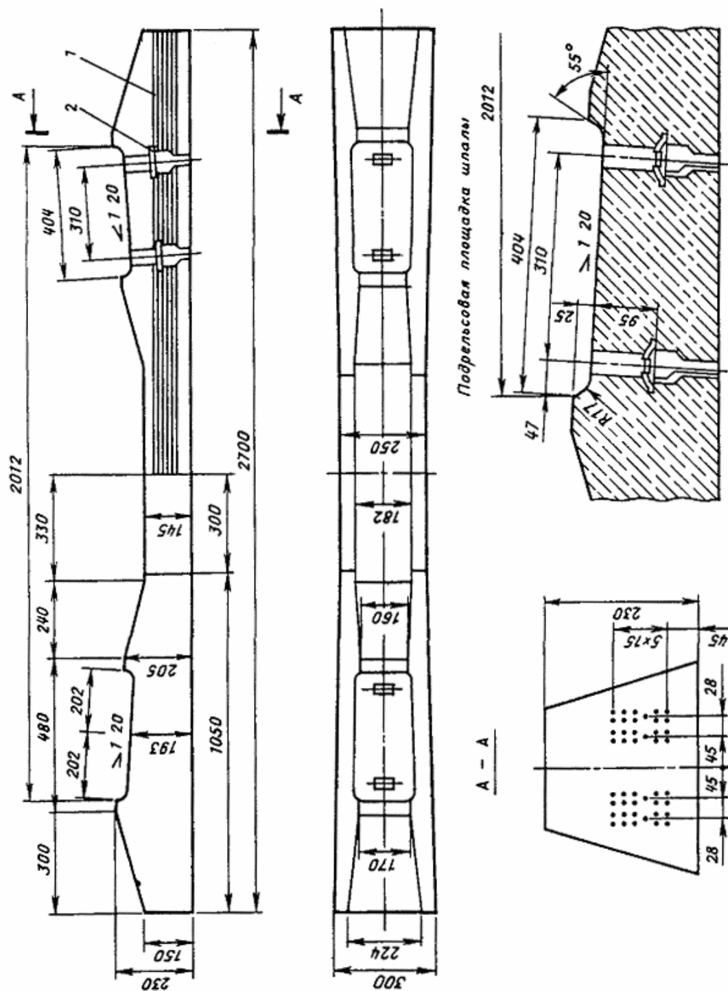
Черт. 20. Шпала железобетонная типа Ш 1-1 по ГОСТ 10629-88
