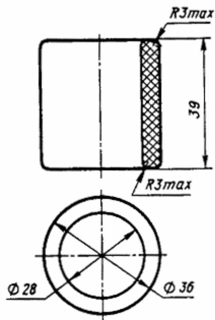
Черт. 147. Втулка В-27
