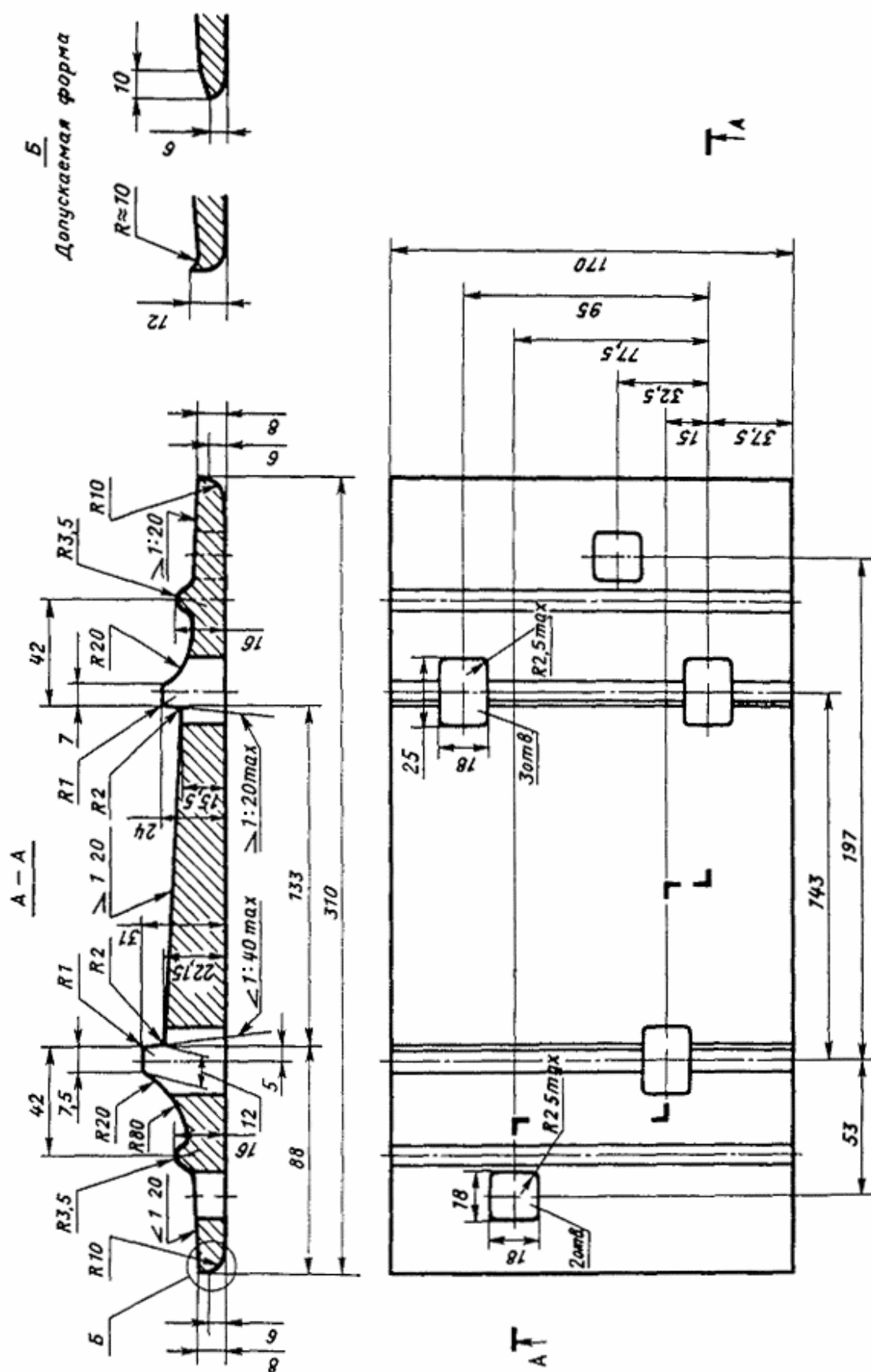
Черт. 66. Подкладка Д50 для костыльного скрепления к рельсам типа Р50 по ГОСТ 12135-75
