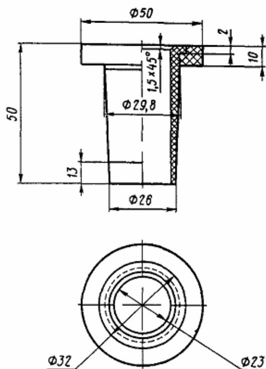
Черт. 114. Втулка изолирующая
